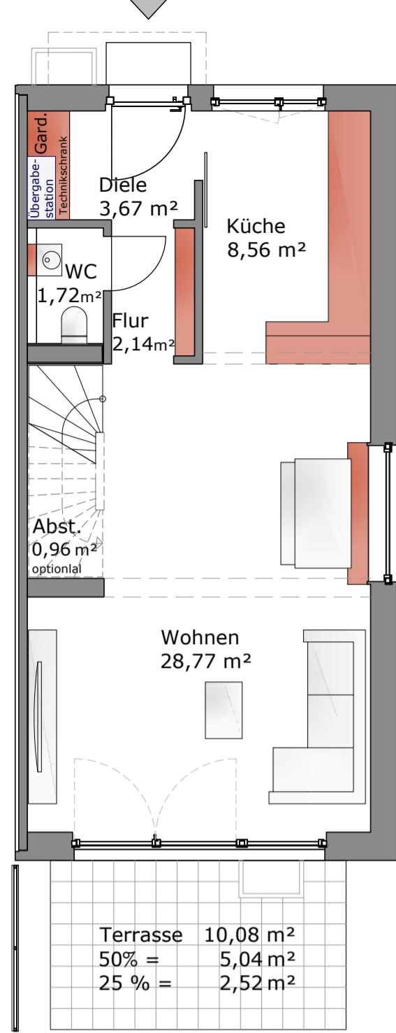
Erdgeschoss
